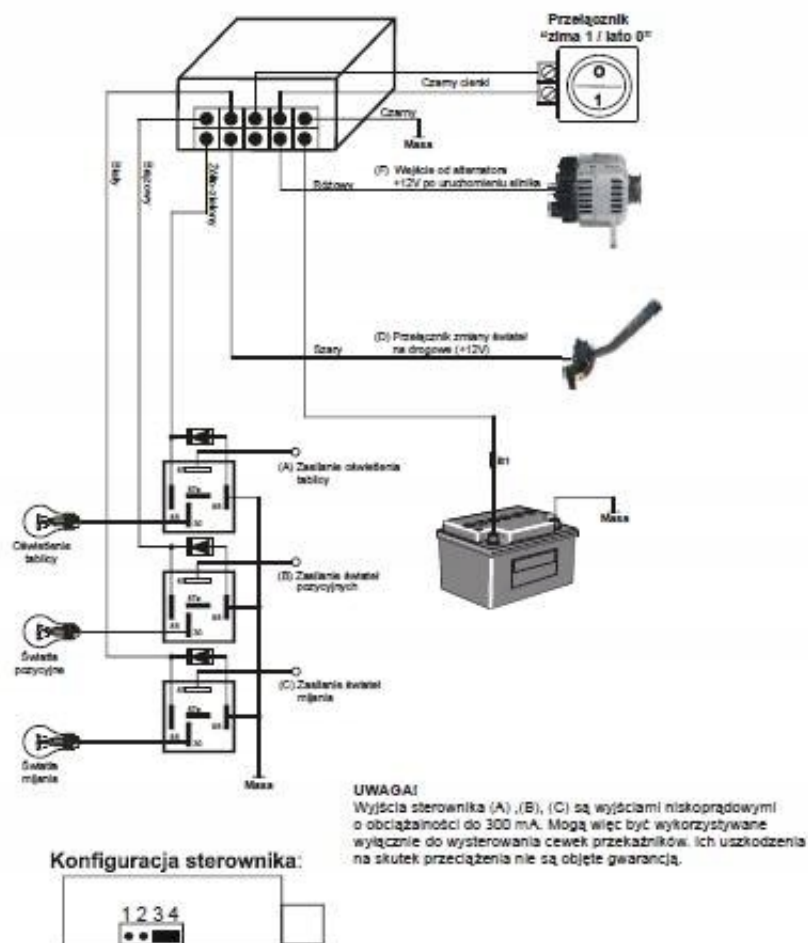
Rys. 2. – Instrukcja montażu dla - Trybu 2:
